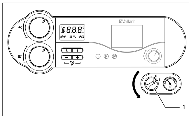
4.18 Вимкнути прилад (на зображенні: atmoTEC/turboTEC plus)
